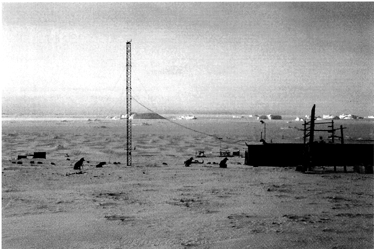
Bild 3: Automatische Synopstation Nr. 04201 des DMI; sendet seit August 1995 stündlich Messdaten über Windrichtung, Windgeschwindigkeit (Mittel und Böen), Temperatur und Luftfeuchtigkeit nach Kangerlussuaq in Südwestgrönland zur Weiterbearbeitung. Standort: Qaanaaq, Nordgrönland, Blickrichtung: S, Höhe: 17 m über Meer. (Adrian Meyer, März 1997)
